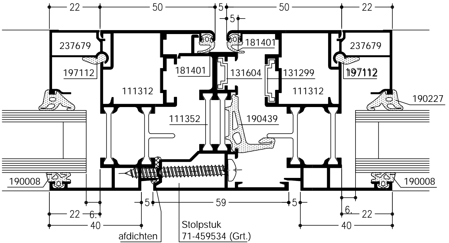
Stolpvlügel met binnen opdek, stolpdetail met opbouwprofiel
