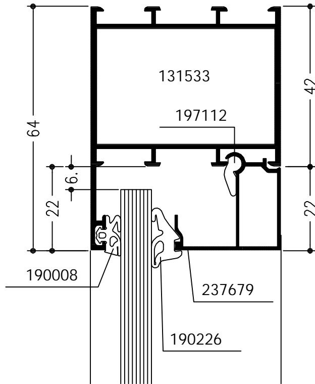
Vlakke deur naar binnendraaiend met vast bovenlicht
