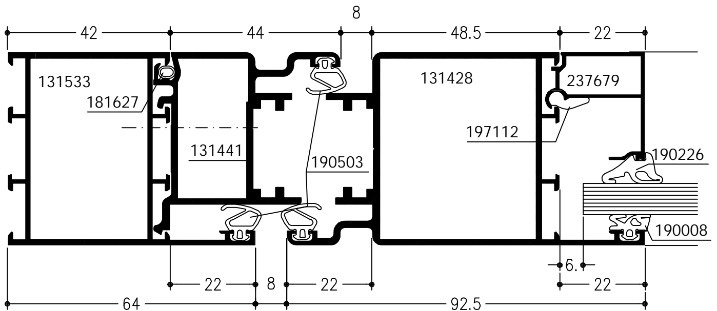
Naar buitendraaiende vlakke deur met combi-kozijn
