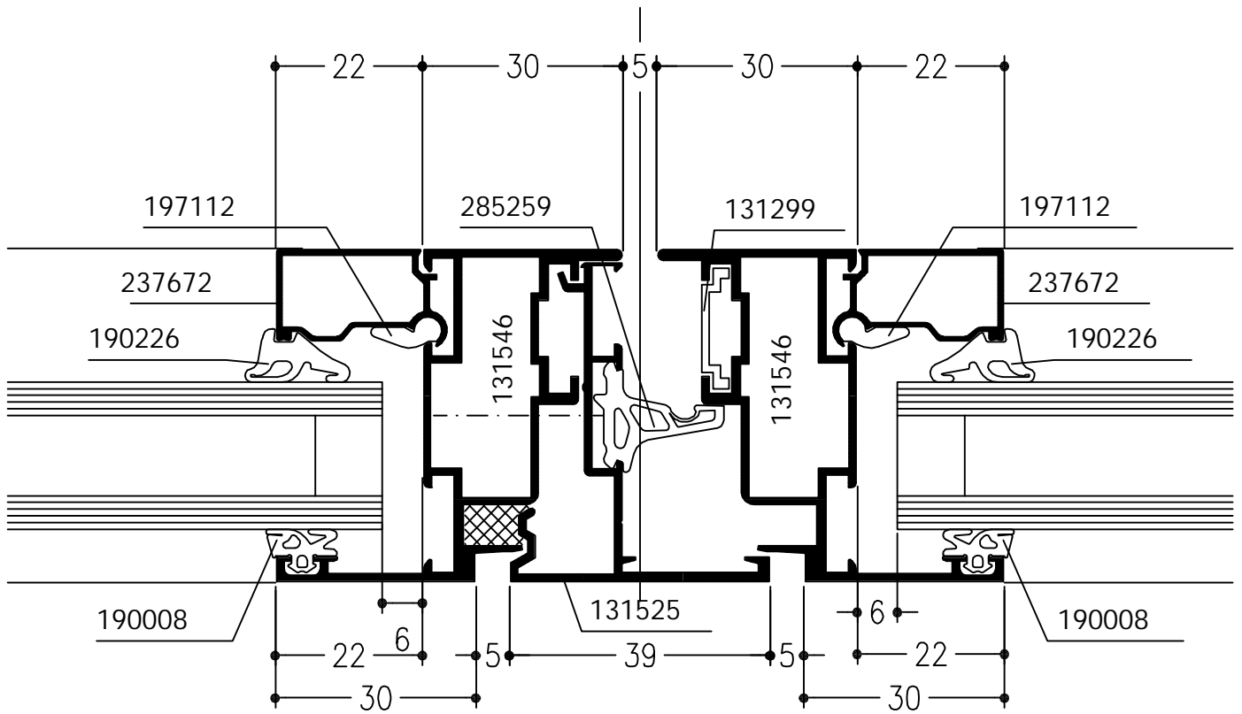
Draairaam, vlakliggend, stolpvluegel
