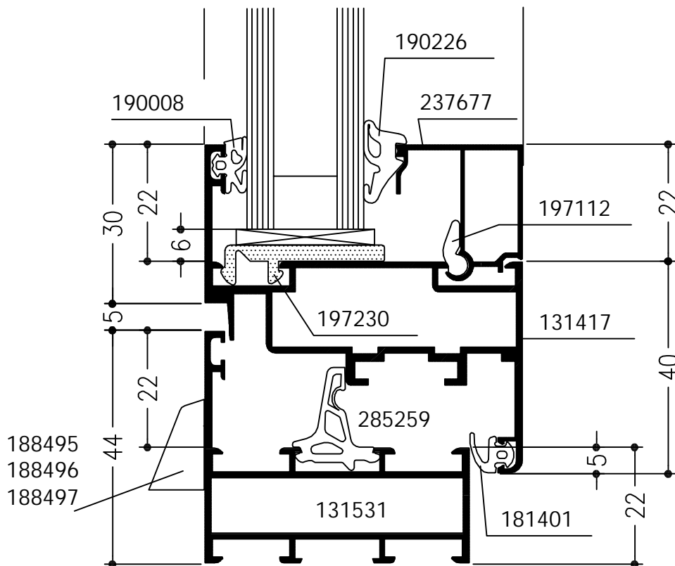
Stolpdraai-, -draaikpraam met opdek
