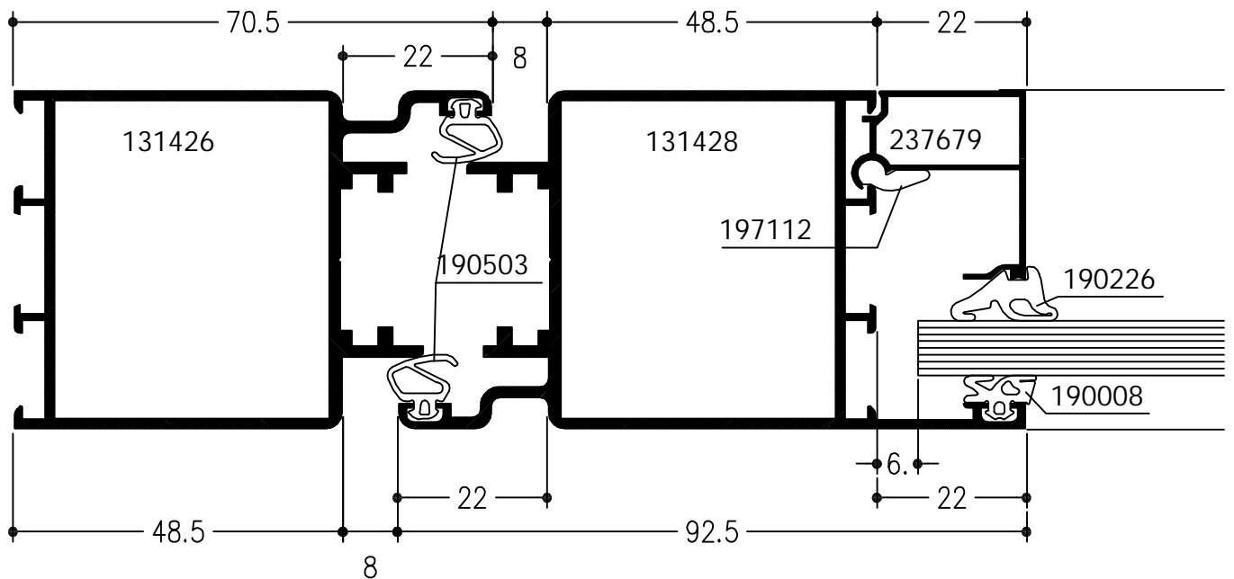
Naar buitendraaiende vlakke deur met speciaal-kozijn
