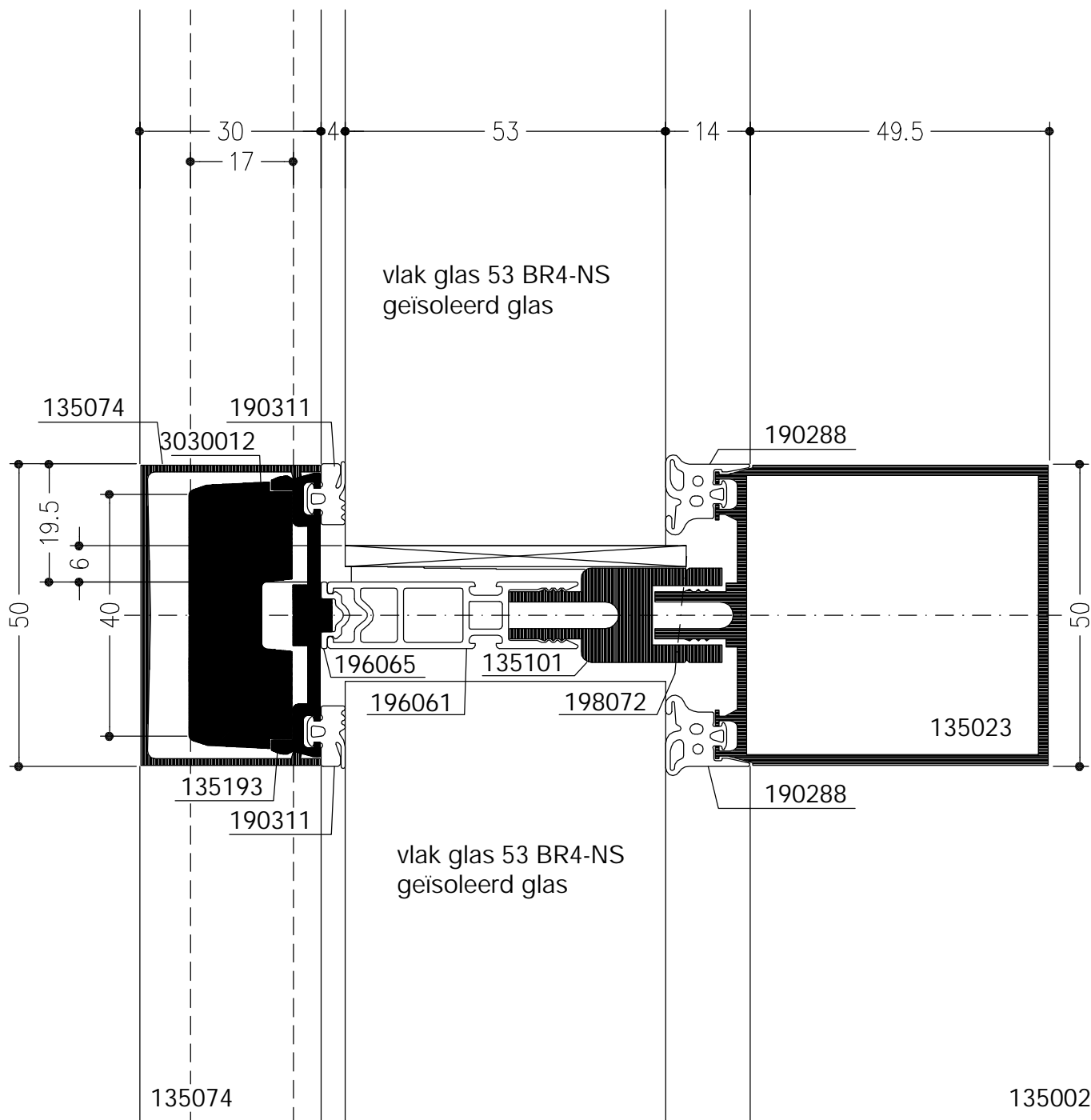
Verticale doorsnede regel E2 met vaste beglazing BR4-NS
