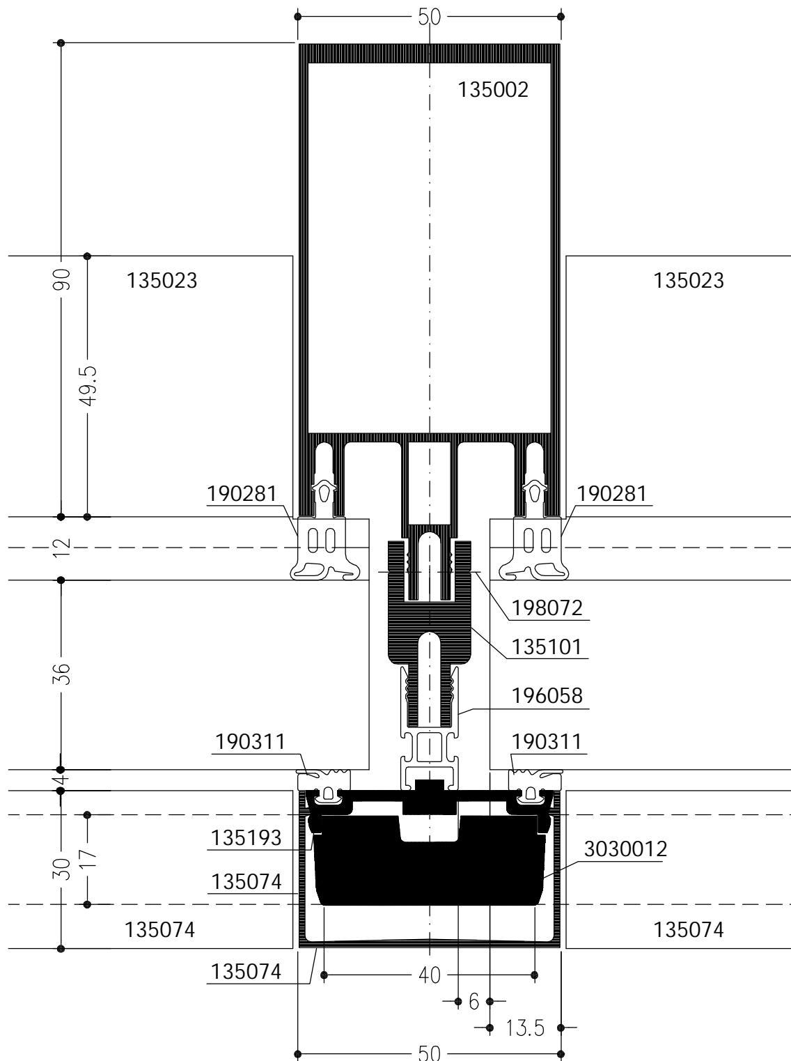
Horizontale doorsnede stijl E1 met vaste beglazing BR4-S
