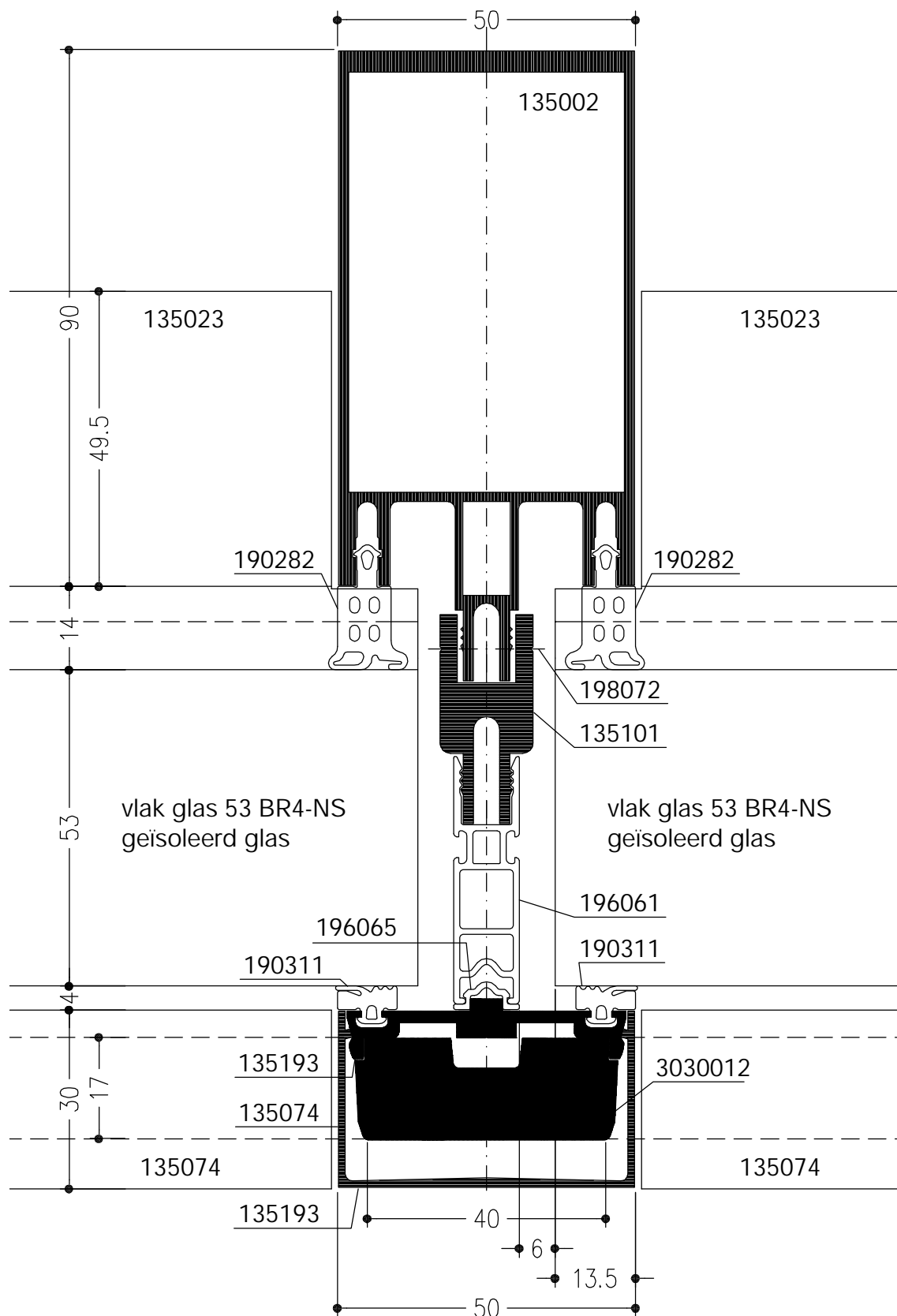
Horizontale doorsnede stijl E1 met vaste beglazing BR4-NS
