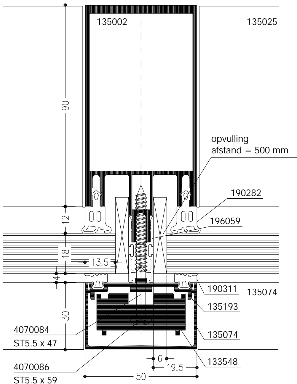
Horizontale doorsnede stijl E1 met enkele beglazing P6B
